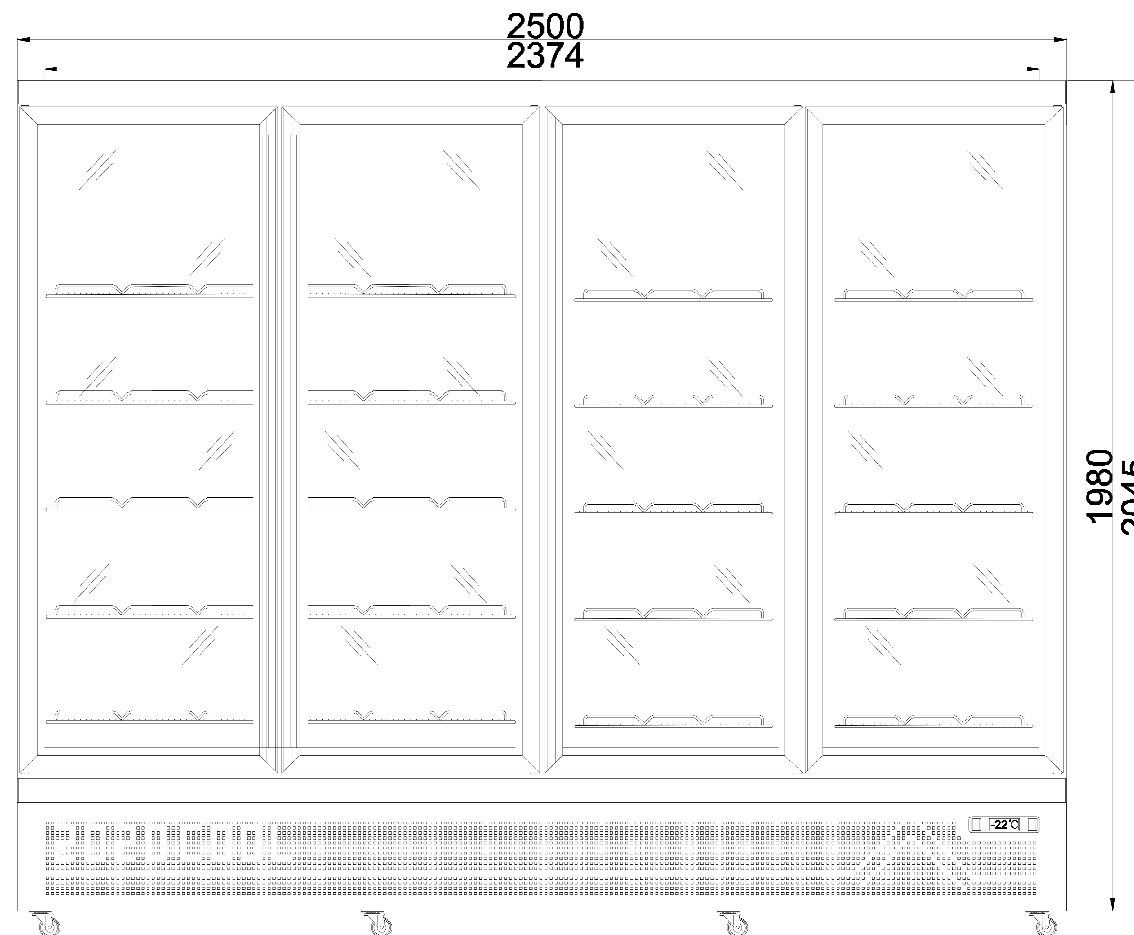
AISLEPRO Four Door Freezer (AISLEPRO 4DF)
